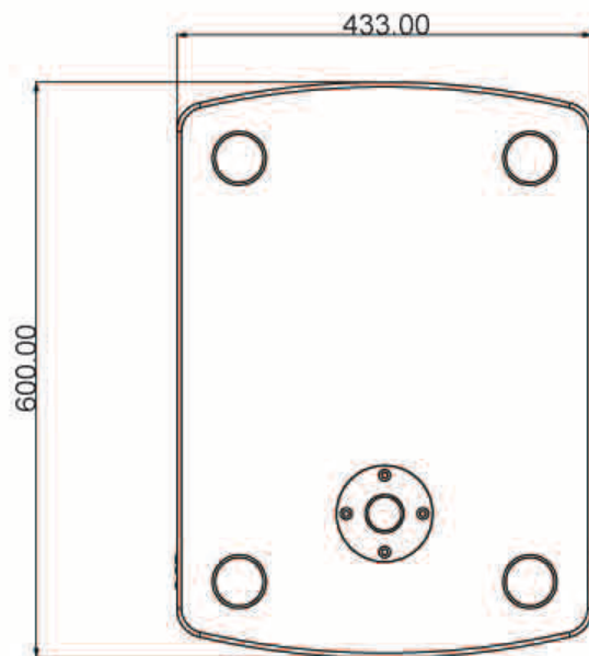
TOP
